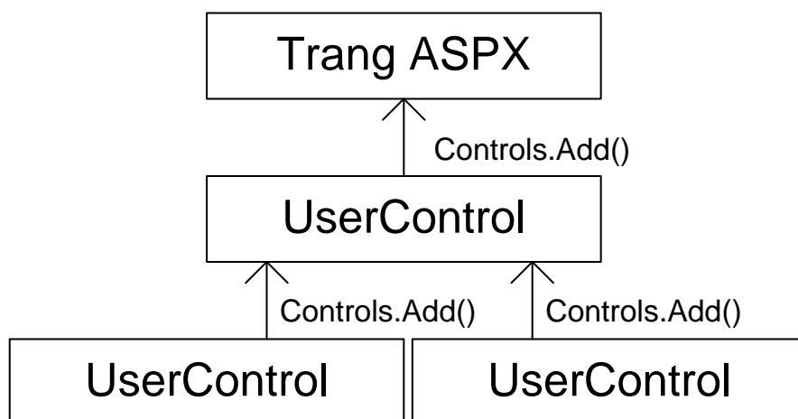
Mô hình kiến trúc tải UserControl động.
