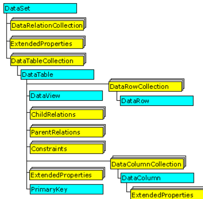
Mô hình Dataset
